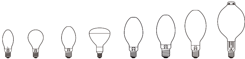
ED17/E26 A23/E26 ED23.5/E39 R40/E26 ED28/E26 ED28/E39 ED37/E39 BT56/E39
